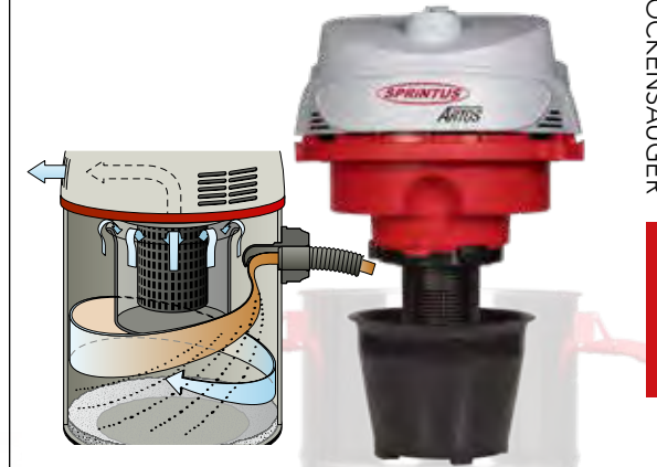
Die Grafik zeigt das patentierte Wasserabscheidesystem mit Zykloneinsatz. Art.-Nr. 116105
