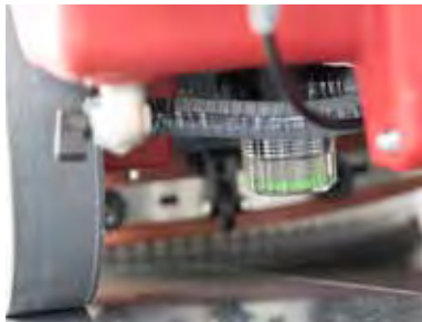
Frischwasser kann restlos und bequem über den Schnellverschluss abgelassen werden.
